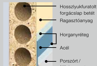
Hosszlyukfuratot forgácslap betét (standard)
