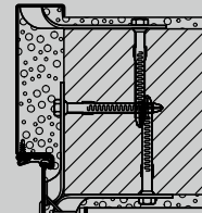
Sarok- és kiegészítőtok Beépítés tiplis rögzítőelemmel
