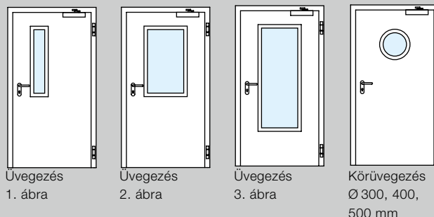
opcionális lekerekített zárású kivitel
