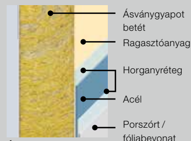
Ásványgyapot betét (opcionálisan) a jobb hőszigetelésért
