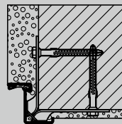
Beépítés tiplis rögzítőelemmel
