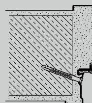
Sarok- és kiegészítőtok rejtett tiplis szereléssel
