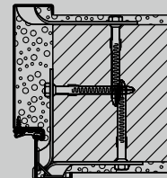
Sarok- és kiegészítőtok Beépítés tiplis rögzítőfülekkel
