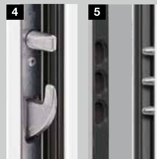
Forgónyelves reteszelés biztonsági csappal
