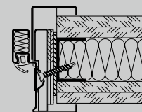
Átlós rögzítés (pórusbeton fal)
