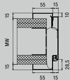
31103 jelű profil, falcolt
