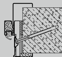
Átlós rögzítés Vario B53 kiegészítőtokkal 2-héjű befoglalótokként (pórusbeton)
