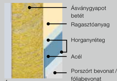
Ásványgyapot betét (opcionálisan) a jobb hőszigetelésért
