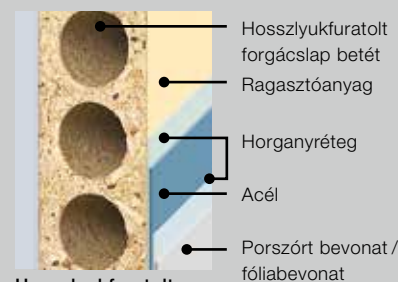
Hosszlyukfuratolt forgácslap betét (standard)
