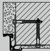
Beépítés tiplis rögzítőfülekkel
