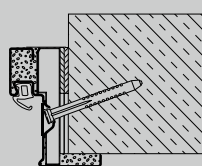
Átlós rögzítés (nem vakolt téglafal / betonfal)
