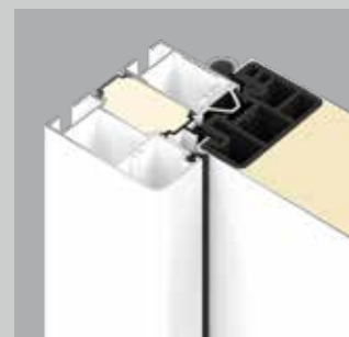
A 65 mm vastag ajtólapal rendelkező MZ Thermo65 többcélú ajtó különösen jó, akár 0,87 \text{ W}/(\text{m}^2 \cdot \text{K}) U_D -értékével elsőosztályú hőszigetelést nyújt.
