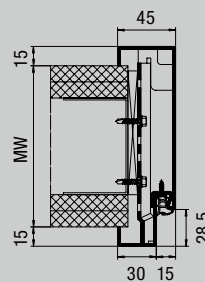
21180 jelű profil, falcolt
