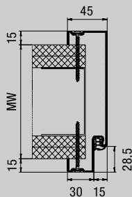
21120 jelű profil, toktükrön keresztüli rögzítés
