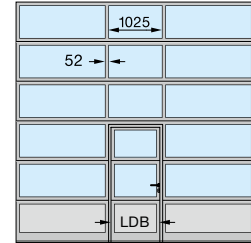
ALR F42, ALR F42 Thermo, ALR 67 Thermo Középre rendezett személybejáró-ajtó
