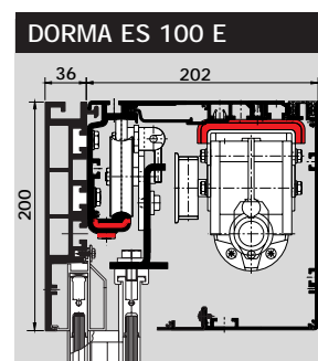
4 Komfort mozgatóegység hangszigetelt motorbeépítéssel, zajmentes futósínnel, és erősebb motorral
