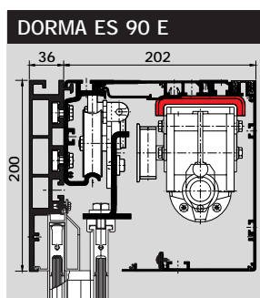
2 Standard mozgatóegység zajcsökkentett futósínnel, hangszigetelt motorbeépítéssel, és erősebb motorral
