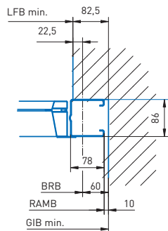
beépítés nyílás mögé
