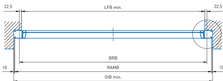
Beépítés nyílás mögé
